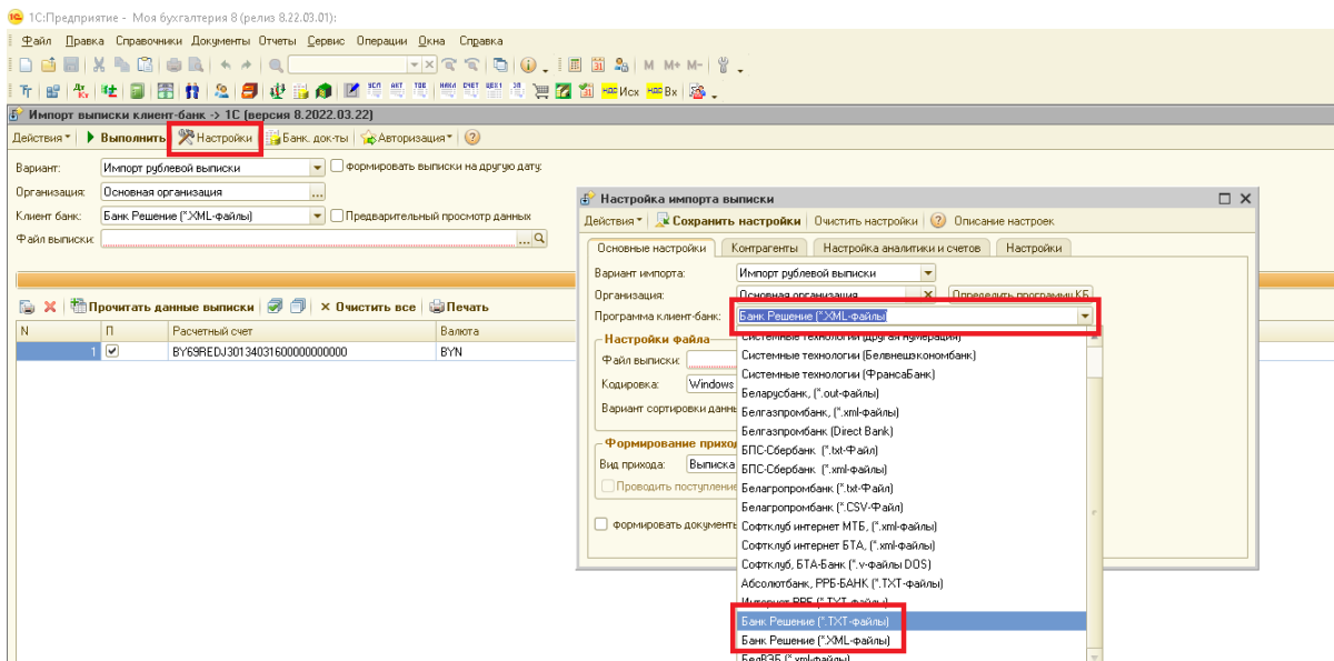
Рисунок 2. Выбор программы клиент-банка для импорта.
