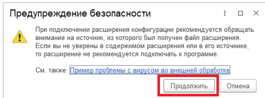
Рисунок 4. Предупреждение безопасности.
