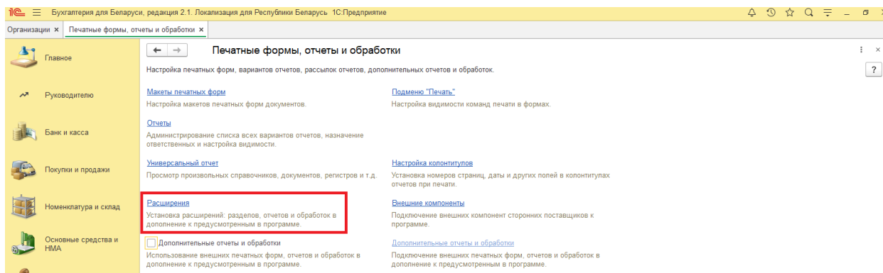
Рисунок 2. Пункт «Расширения».
