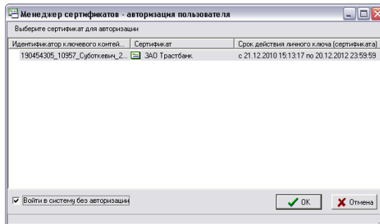
Рисунок 1 – Авторизация пользователя
