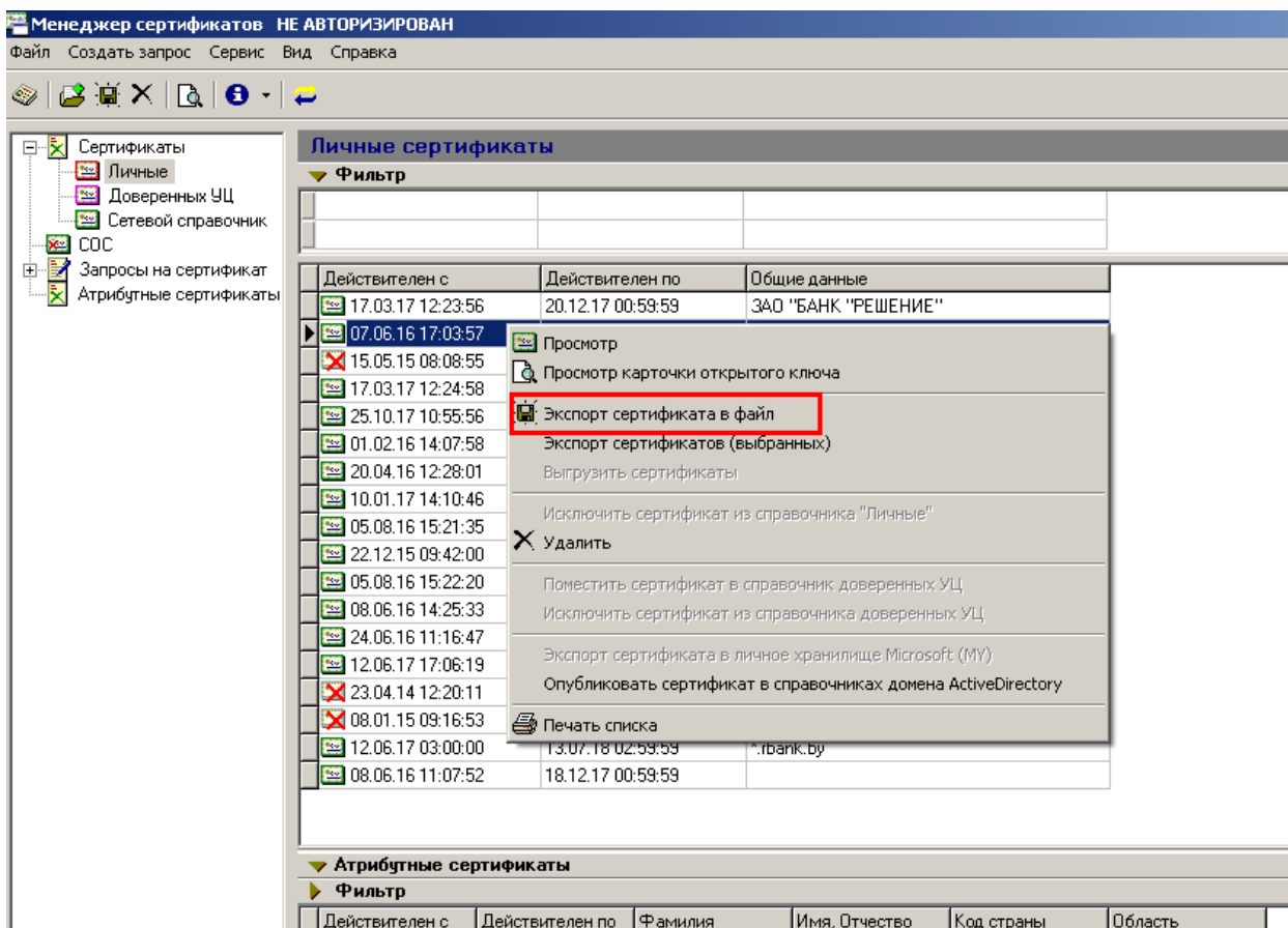
Рисунок 2 – Список сертификатов
